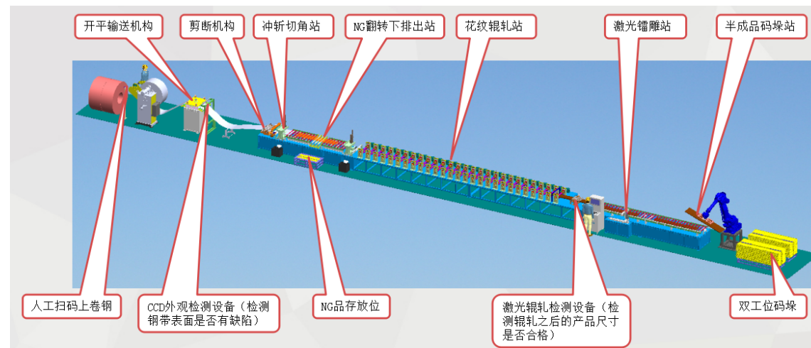
门框花纹数字化生产线
