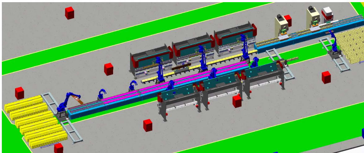
非标门框柔性数字化生产线
