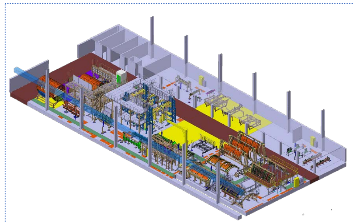
中机身装配生产线
